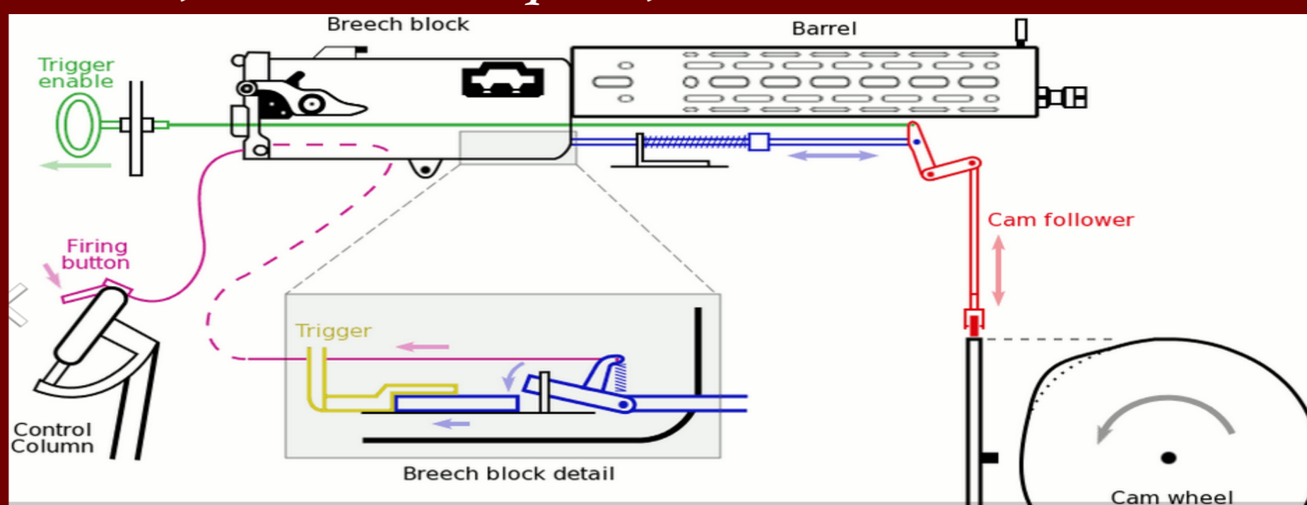
Diagramme du système de synchronisation Fokker. Tirer la poignée verte abaisse la bielle rouge sur la roue à une came associée à l'axe de l'hélice. Lorsque la came soulève la bielle, la tige bleue est abaissée contre la gâchette. Ainsi, lorsque le bouton de tir violet est pressé, la tige bleue pousse la gâchette permettant à la mitrailleuse de tirer.
